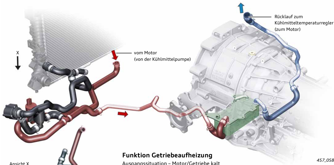
Ansicht X
