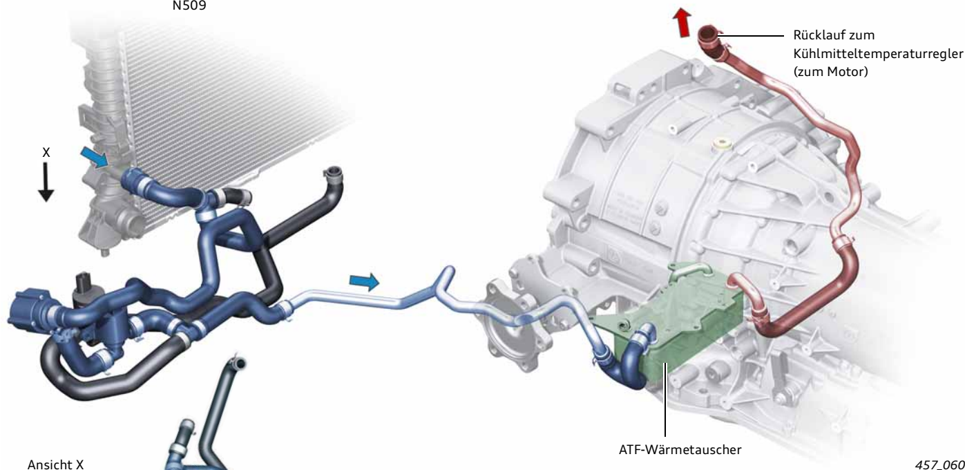
Ansicht X
