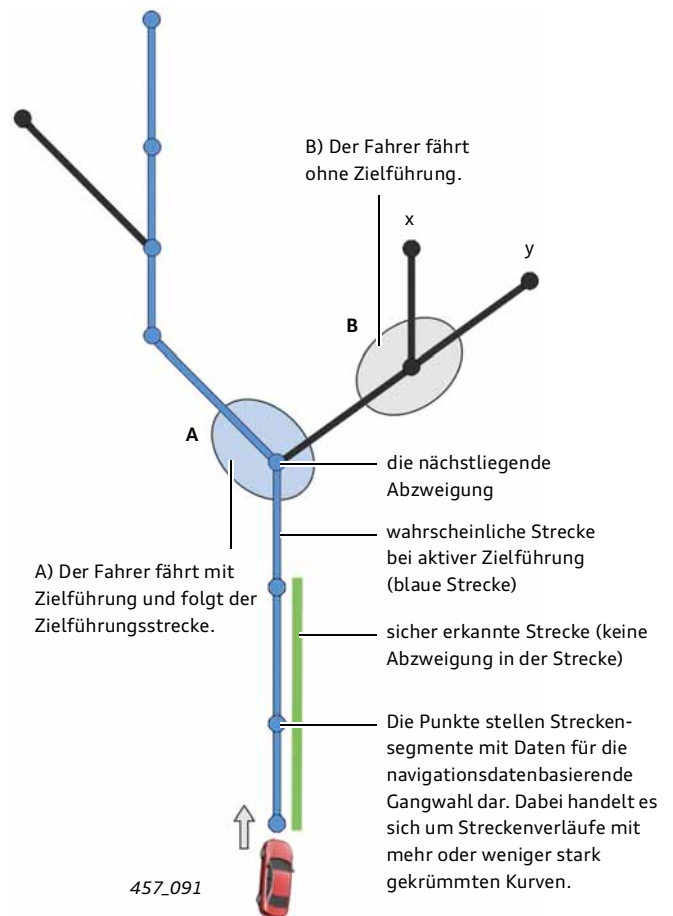
Schematische Darstellung des vorausschaubaren Streckenbereichs bei aktiver Zielführung, „vorausschaubarer Streckenbaum“
