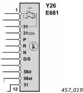
Funktionsplan (Ausschnitt)
