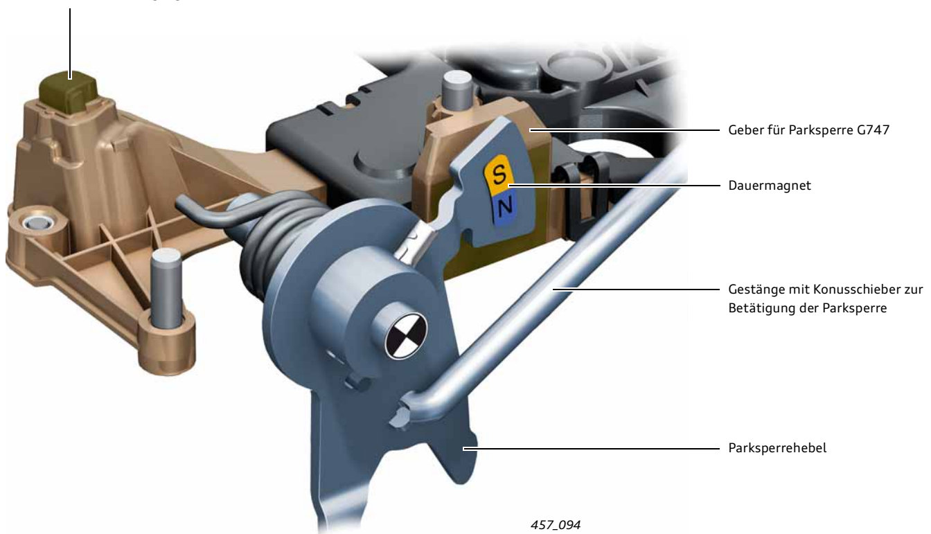
Geber für Getriebeeingangsdrehzahl G182
