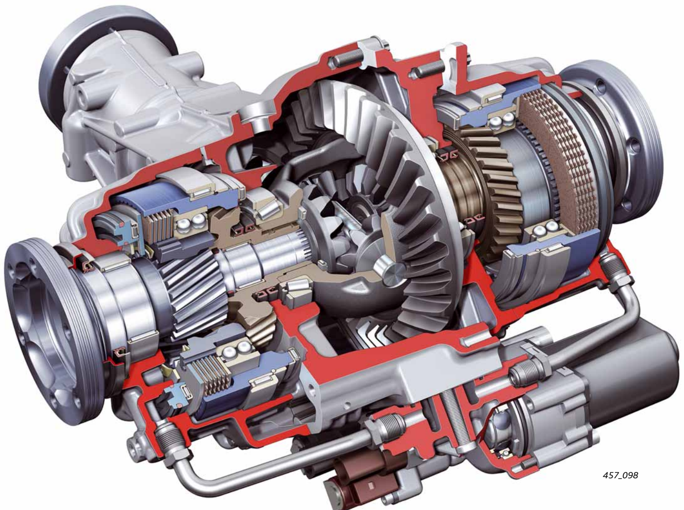
Achsantrieb hinten OBF/Sportdifferenzial (bis 700 Nm)
