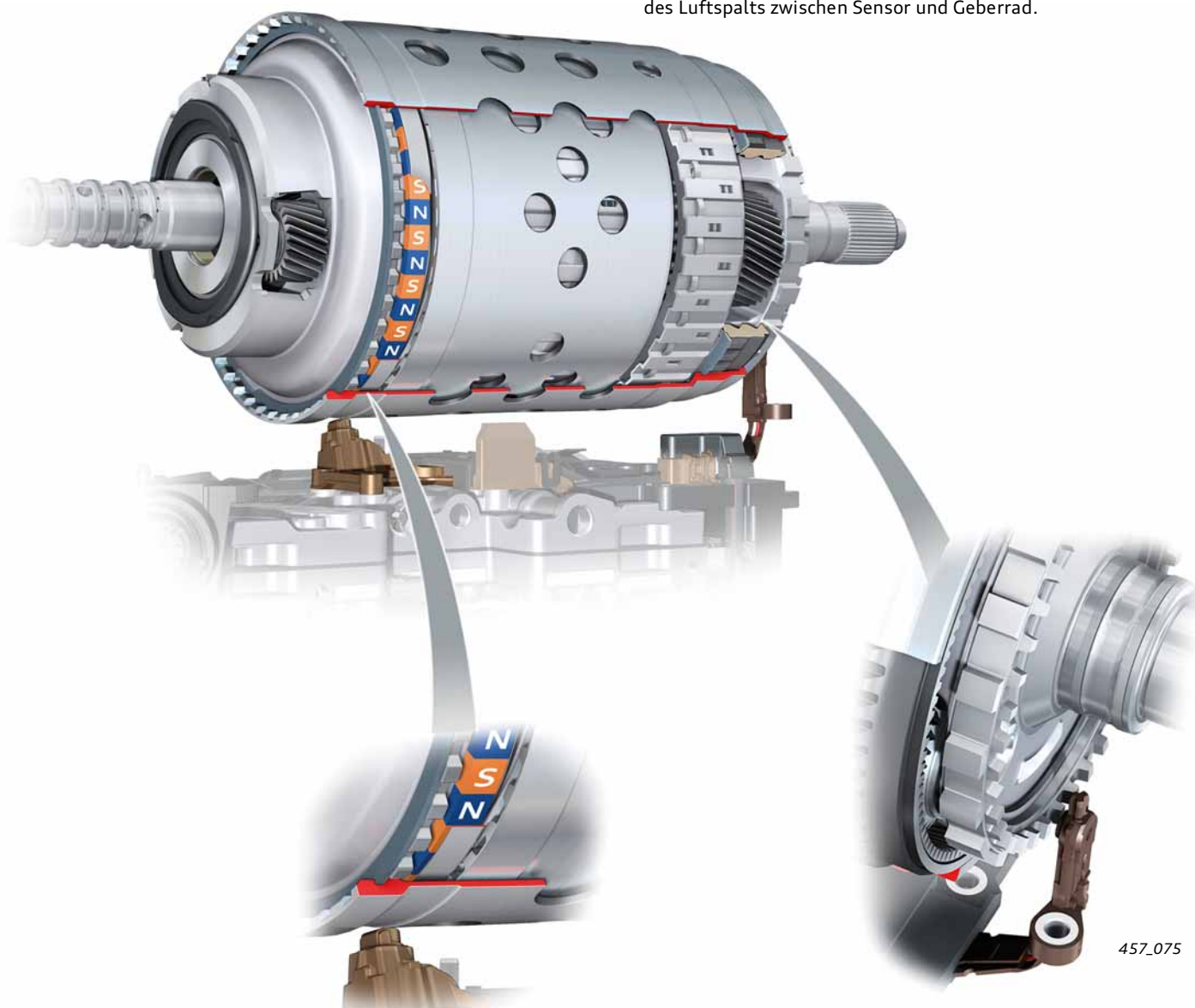
Geber für Getriebeeingangsdrehzahl G182
